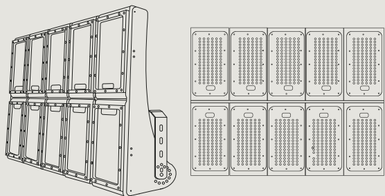
Proyectores High Bay IP66 Sport Arena Referencias de 8, 10 y 12 Modulos.
